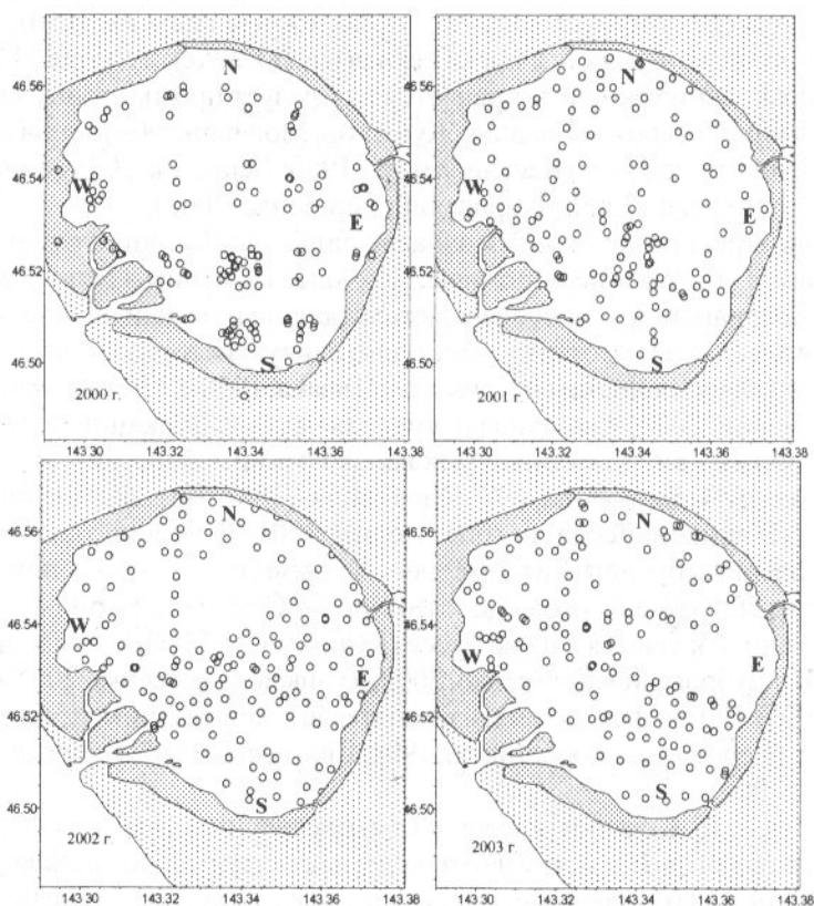
Рис. 1. Схемы водолазных станций, выполненных в период 2000–2003 гг. в лагуне Буссе: ○ – точки водолазных станций
