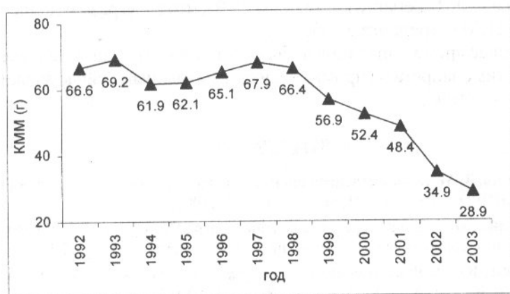
Рис. 4. Динамика средней массы кожного-мышечного мешка трепанга лагуны Буссе
