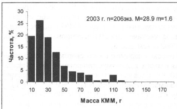
Рис. 3. Массовый состав трепанга лагуны Буссе в летний период 2000–2003 гг.
