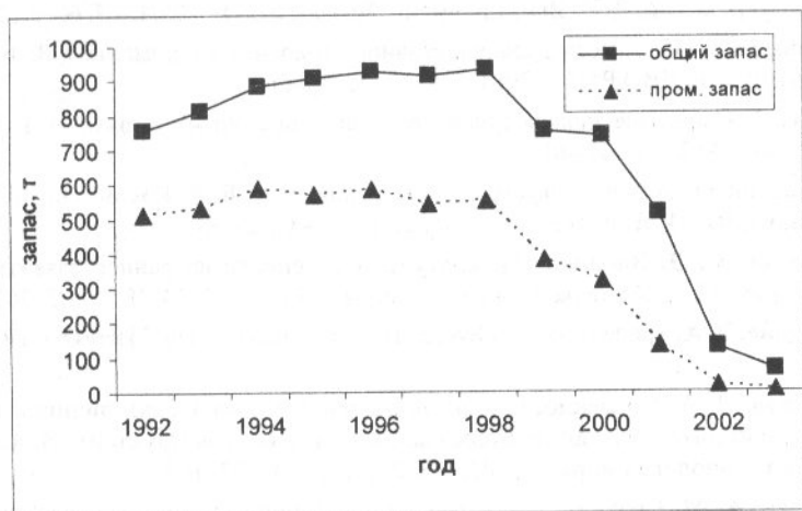
Рис. 5. Динамика общего и промыслового запасов дальневосточного трепанга в лагуне Буссе
