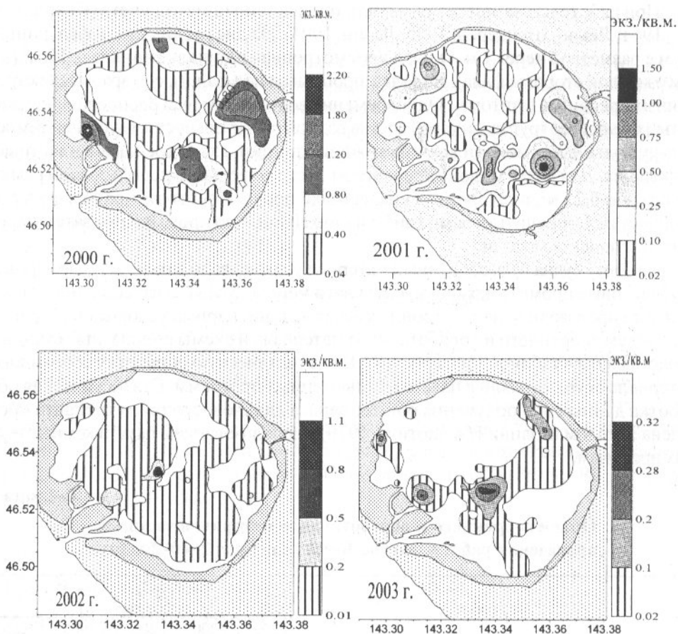
Рис. 2. Схемы распределения дальневосточного треска в лагуне Буссе по результатам исследований 2000–2003 гг.
