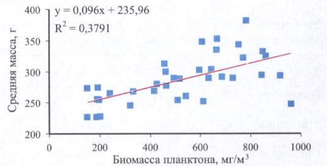
Рис. 5. Средняя длина и масса 4–10-годовиков корфо-карагинской сельди в зависимости от биомассы зоопланктона
