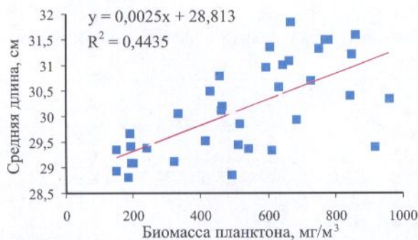
Рис. 5. Средняя длина и масса 4–10-годовиков корфо-карагинской сельди в зависимости от биомассы зоопланктона
