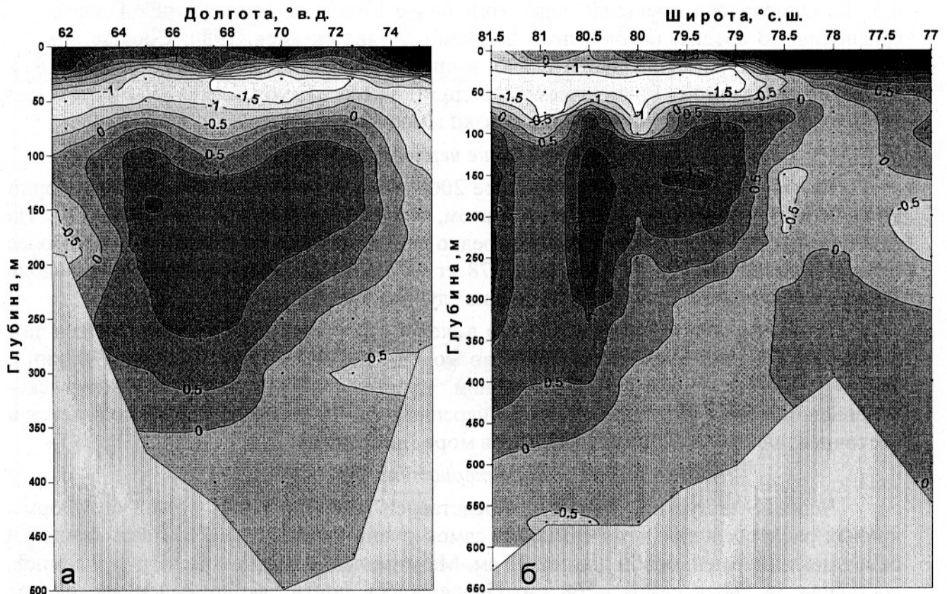
Рис. 4. Вертикальное распределение температуры, °С на условных разрезах К-1 (а) и К-2 (б) желоба Святой Анны. Fig. 4. Vertical distribution of temperature (°С) in the sections К-1 (а) and К-2 (б) in the Svyataya Anna Trough.
