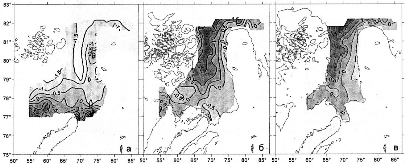
Рис. 3. Распределение температуры, °С на горизонте 50 (а), 200 (б) и 300 (в) м в августе-сентябре 2008 г. Fig. 3. Temperature, °С at 50 (a), 200 (б) and 300 (в) m depth in the August-September 2008.
