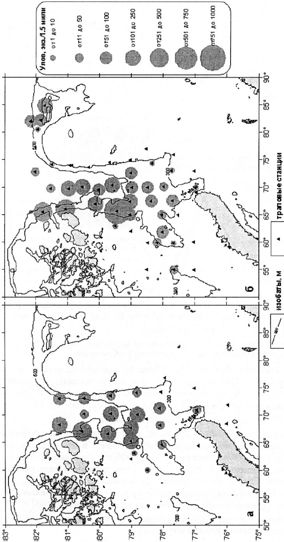
Рис. 6. Распределение уловов черного палтуса по данным НИС «Фридьоф Нансен» в августе-сентябре 2007 г. (а) и М-0075 «Обва» в августе-сентябре 2008 г. (б)
