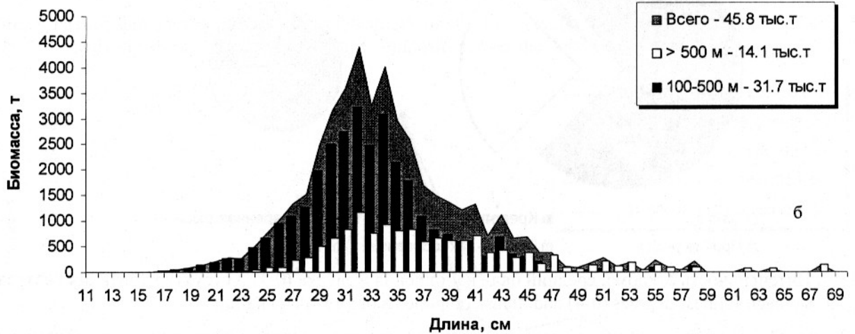
Рис. 10. Распределение численности (а) и биомассы (б) черного палтуса различной длины по диапазонам глубин.
