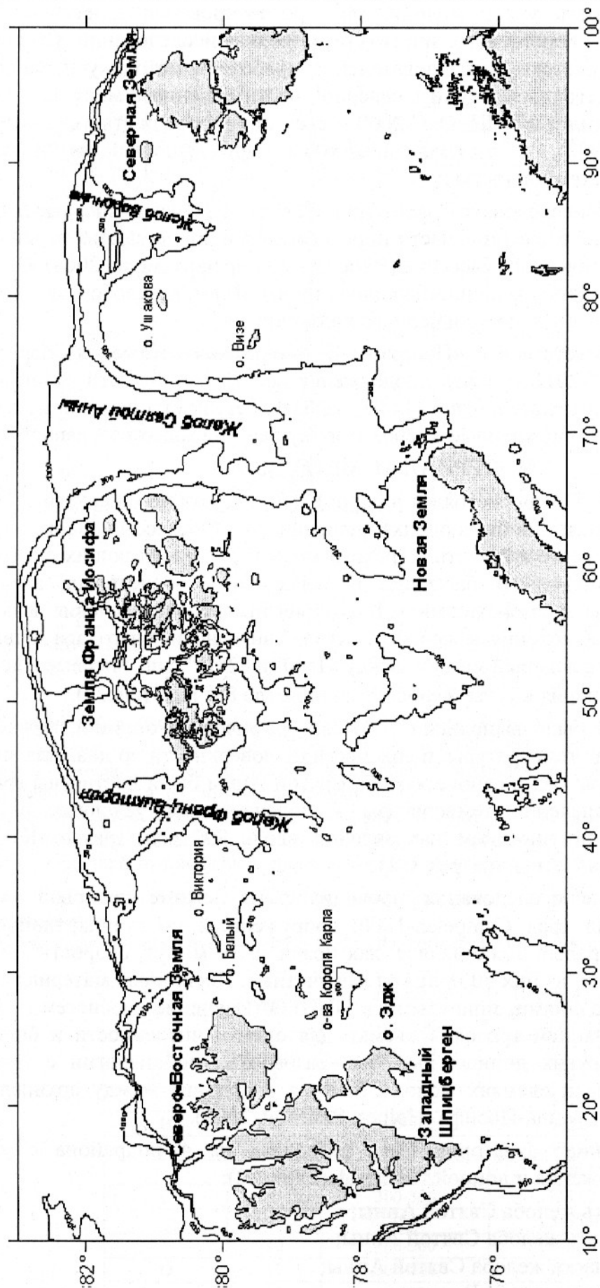
Рис. 1. Схема северной окраины шельфа Баренцева и Карского морей. Fig. 1. Scheme of the northern borderland of the Barents and Kara Seas slopes.
