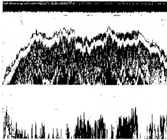
Рис.22. Эхограмма записи ламинариевых водорослей, эхолот “Шкипер-607”, диапазон 0-20 м, режим “белая линия”, диапазон расширения 2 м (Пестриков, 1992)
