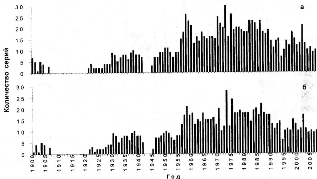
Рис. 2. Количество серий наблюдений за температурой (а) и соленостью (б) воды на разрезе «Кольский меридиан» в 1900-2007 гг. (www.pinro.ru).
