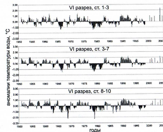
Рис. 4. Среднемесячные аномалии температуры воды в слое 0-200 м на станциях VI разреза Баренцева моря (Матишов и др., 2000 а; Терещенко, 1999). В правой части диаграммы добавлены аномалии температуры с 1999 по 2005 гг., рассчитанные в данной работе.
