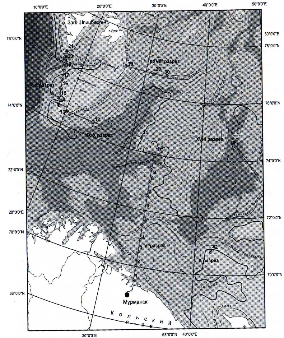
Рис. 3. Станции стандартных разрезов, выполненные в экспедициях ММБИ в 1999-2005 гг. Батиметрическая основа по (Matishov, 1997). Схема поверхностных течений по (Танцора, 1959; Новицкий, 1961)
