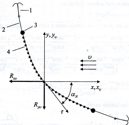
Рис. 13. Характеристики ставной сети в потоке:
