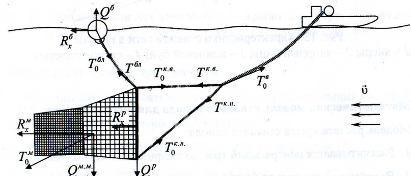
Рис. 12. Специализированный подхват для лова медузы
