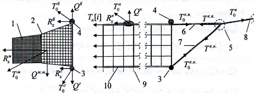
Рис. 11. Устройства для лова медуз (Бородин, Осипов, 2002): 1 – мешок; 2 – мотня; 3 – груз; 4 – буй; 5 – соединение верхнего и нижнего кабелей с ваером; 6 – кабель верхний; 7 – кабель нижний; 8 – ваер; 9 – распределенная загрузка по нижней подборе; 10 – крыло
