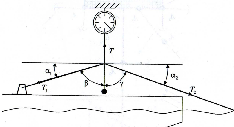
Рис. 15. Схема измерения натяжения T и углов \alpha_1 , \alpha_2 ваера
