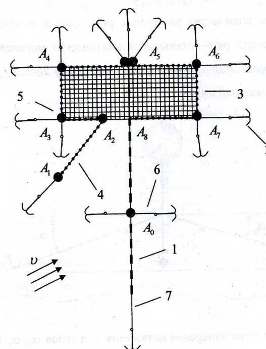
Рис. 14. Ставной невод для лова медуз: 1 – крыло; 2 – якоря; 3 – ловушка; 4 – открылок; 5 – буй; 6 – оттяжки; 7 – центральный трос
