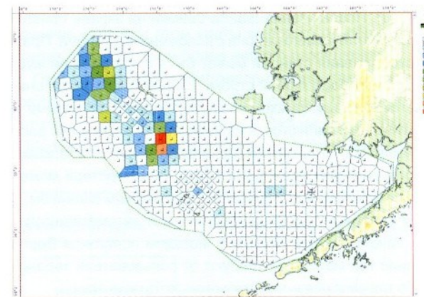
Полигоны Вороного
