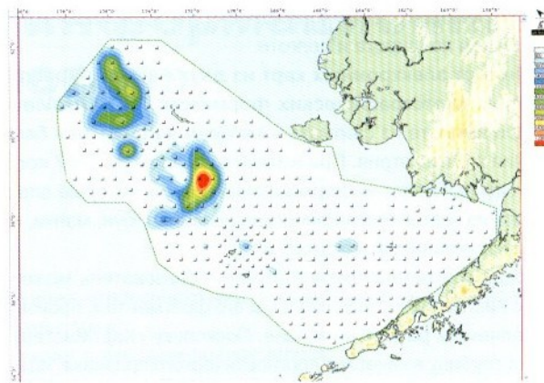
Профессиональный кригинг
