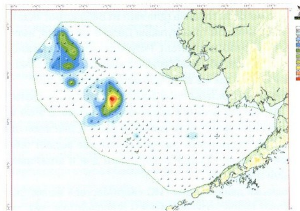
Автокригинг
