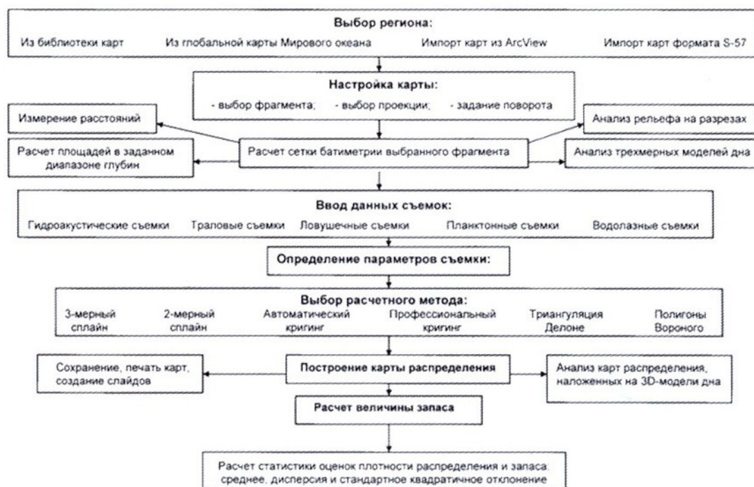
Рис. 1. Функциональная схема ГИС «КартМастер»
