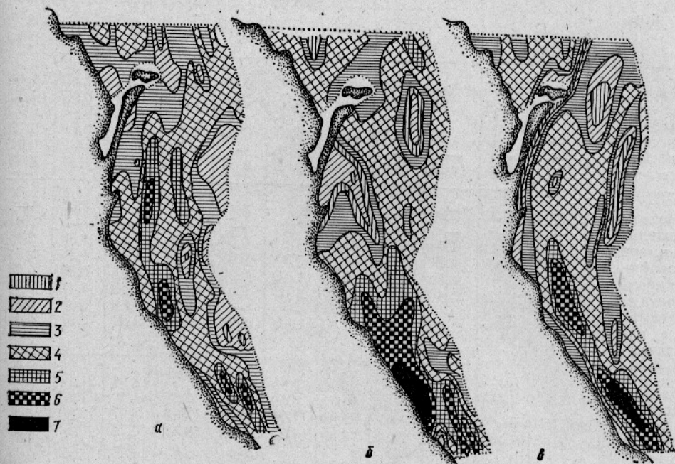
Рис. 1. Распределение общей биомассы бентоса в 1960 г.:
