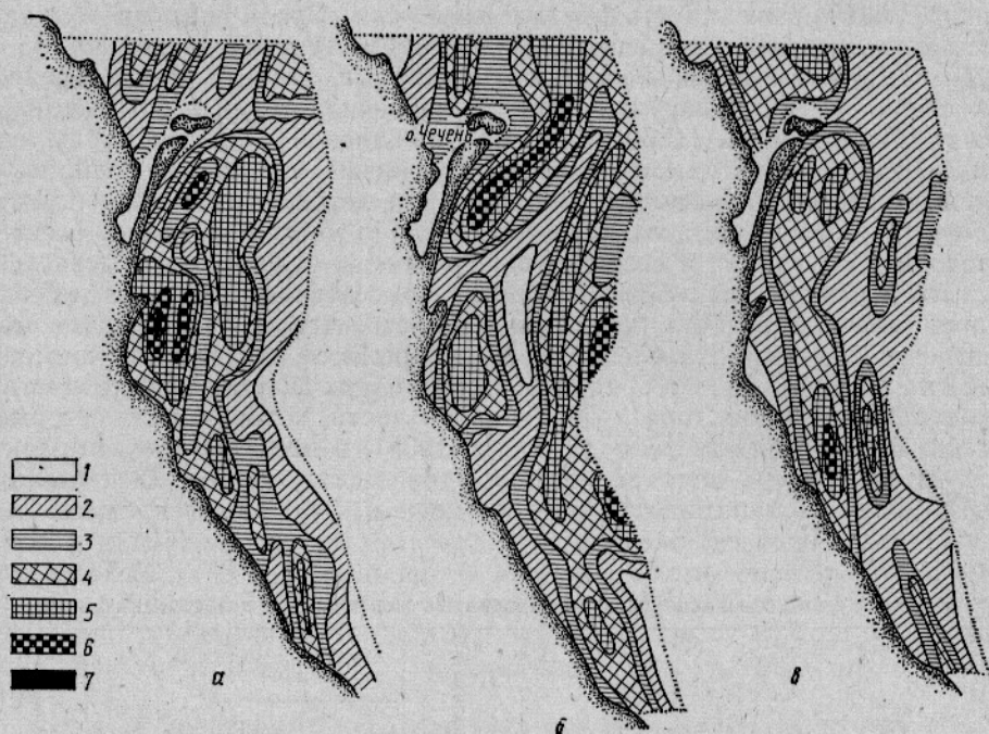
Рис. 3. Распределение биомассы Nereis diversicolor ;
