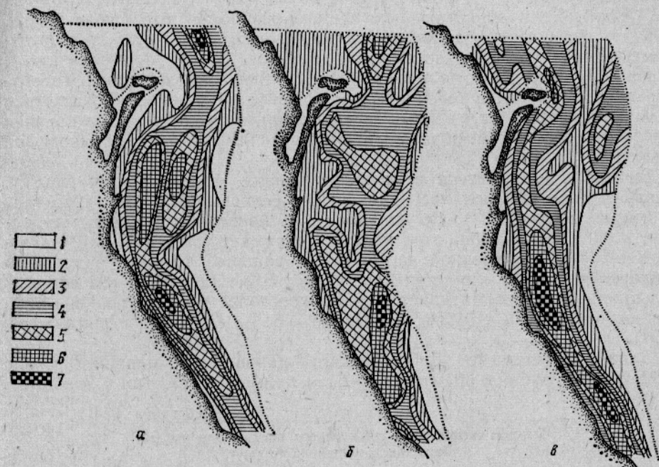
Рис. 2. Распределение биомассы Abra ovata :
