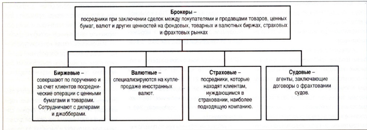
Рис. 5. Функции брокеров
