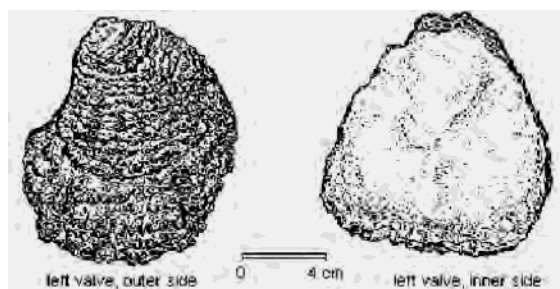
Рис. 1. Типичный экземпляр черноморской устрицы Ostrea edulis (Linnaeus, 1758)
