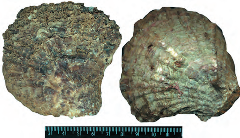
Рис. 8. Экземпляр черноморской устрицы с вертикальной скалы (Судакский залив, 1985 г., глубина 4 м, шкала в см)
