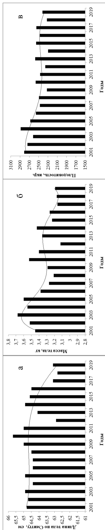
Рис. 3. Динамика длины (а), массы тела (б) и плодовитости (в) североохономорской кеты в начале XXI в.
