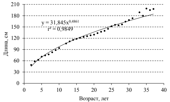
Рис. 1. Кривая линейного роста амурского осетра
